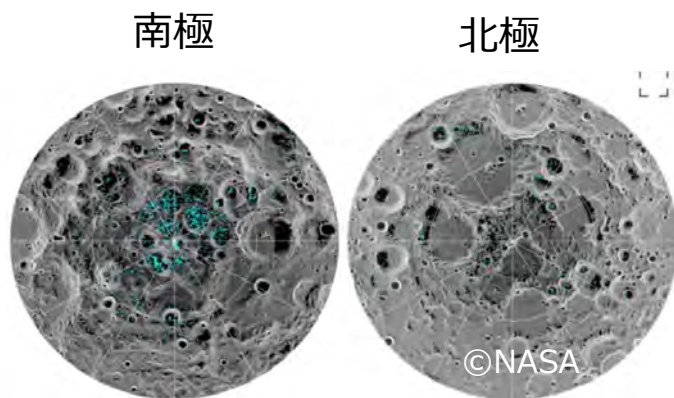
月極における水の分布。クレーターの影・地軸の傾きで水資源が氷の形で残っている。(水色部分)
