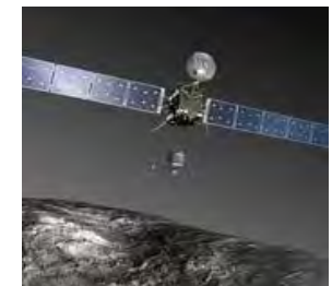
Rosetta
