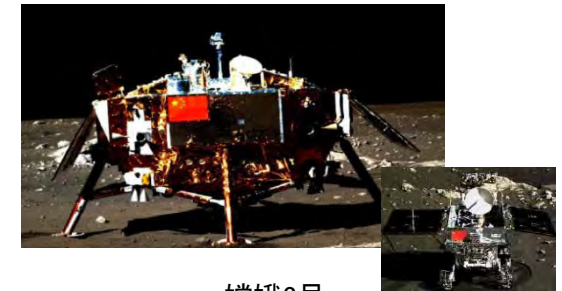
嫦娥3号
