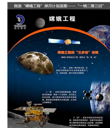
嫦娥計画
