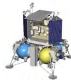
Luna-25 (Luna-Glob) 2016
