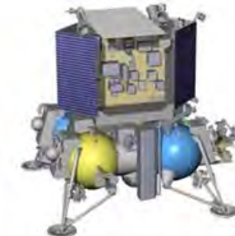
Luna-27 (Luna-Resurs 1) 2019
