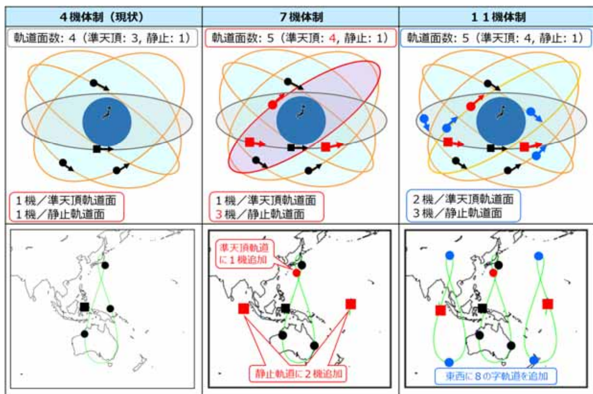
図 準天頂衛星システム「みちびき」の軌道追加、地上投影イメージ
