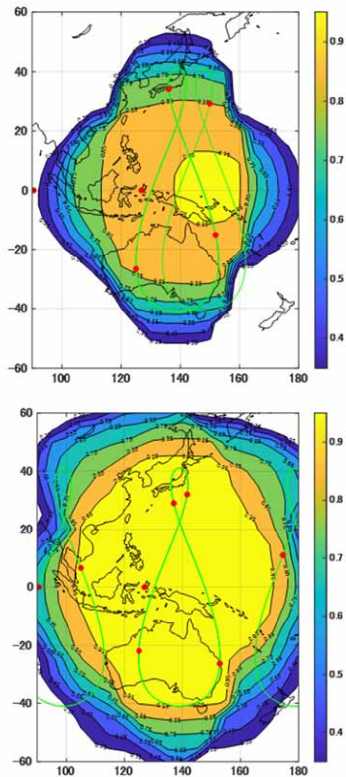
図 HDOP2.6 が得られる時間率分布の違いの目安(上:7機、下:11機)
