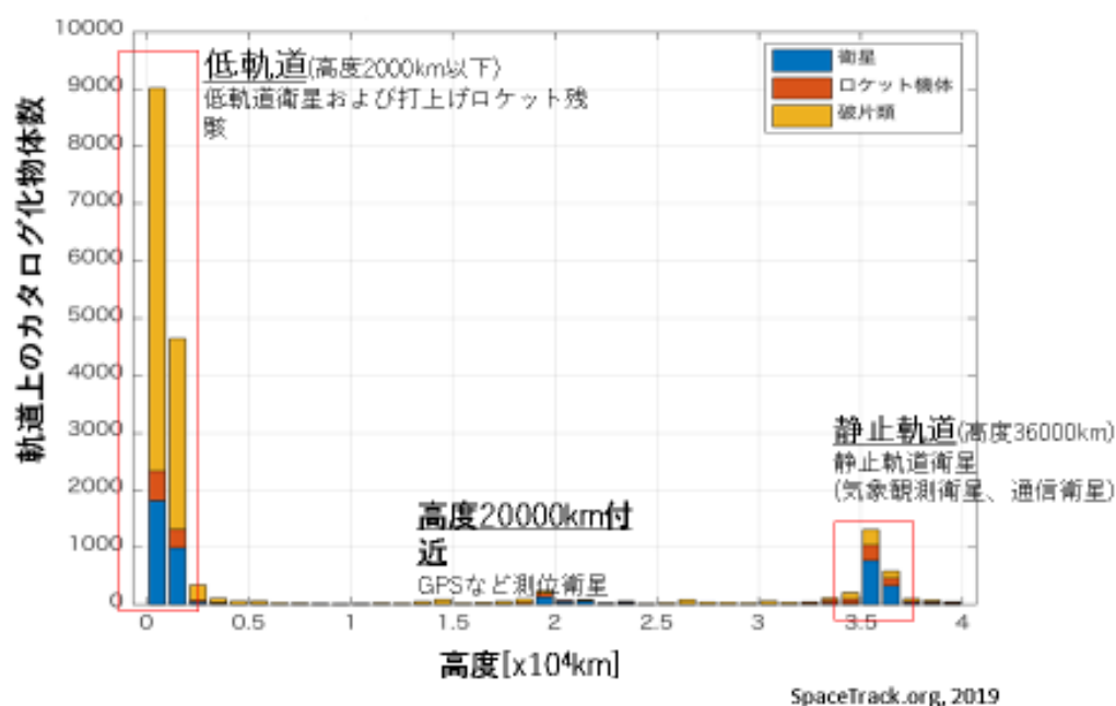
図2 軌道上の衛星分布現状
